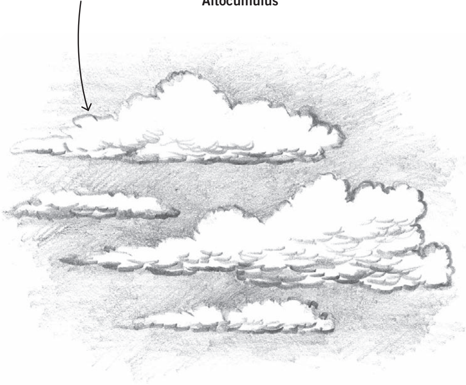
Alto cumulus
