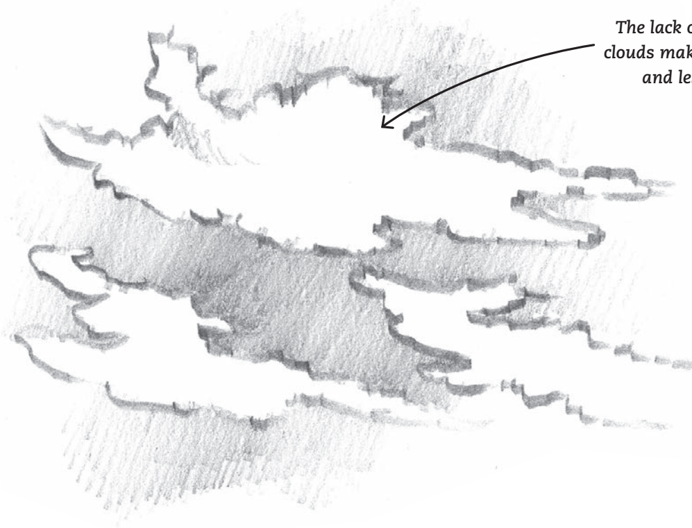
Cirrus Fibractus
