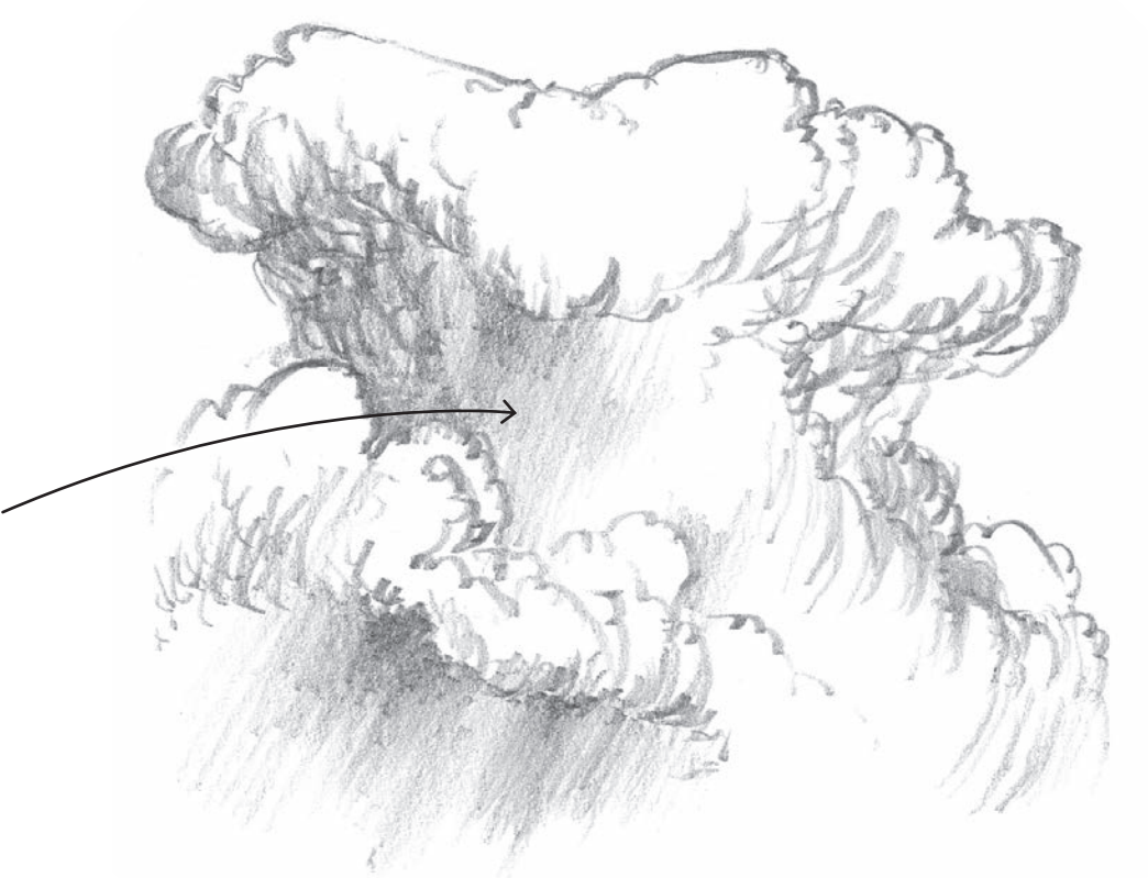
Cumulonimbus
